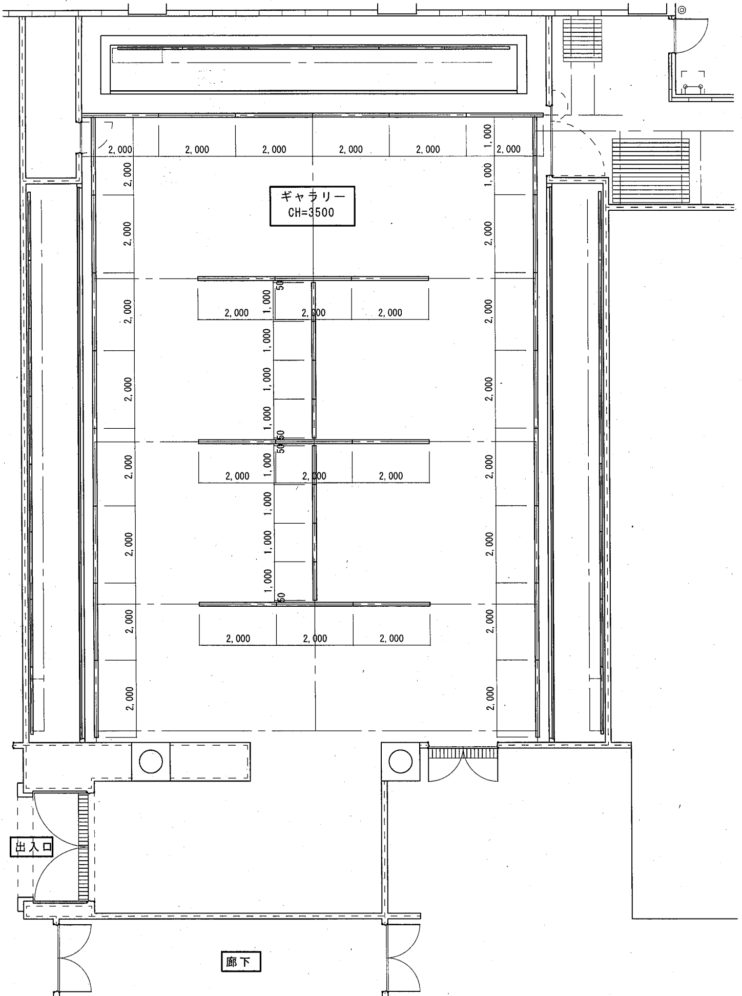
ギャラリー 平面図 S=1/100
